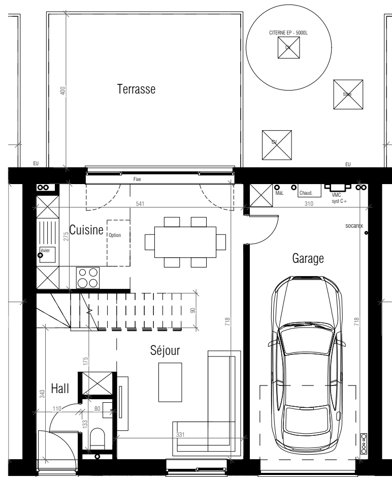
REZ-DE-CHAUSSÉE
